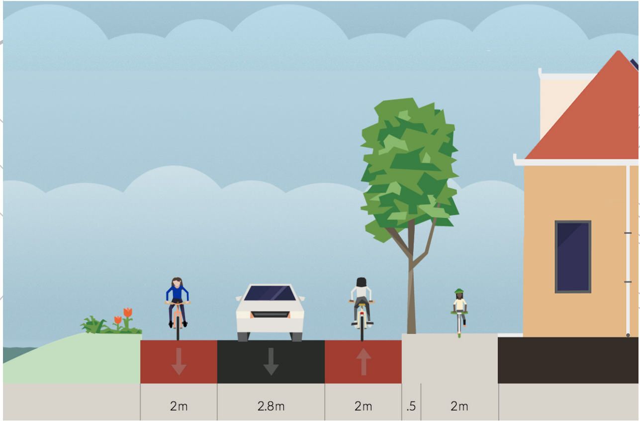
DWARSDOORSNEDE
