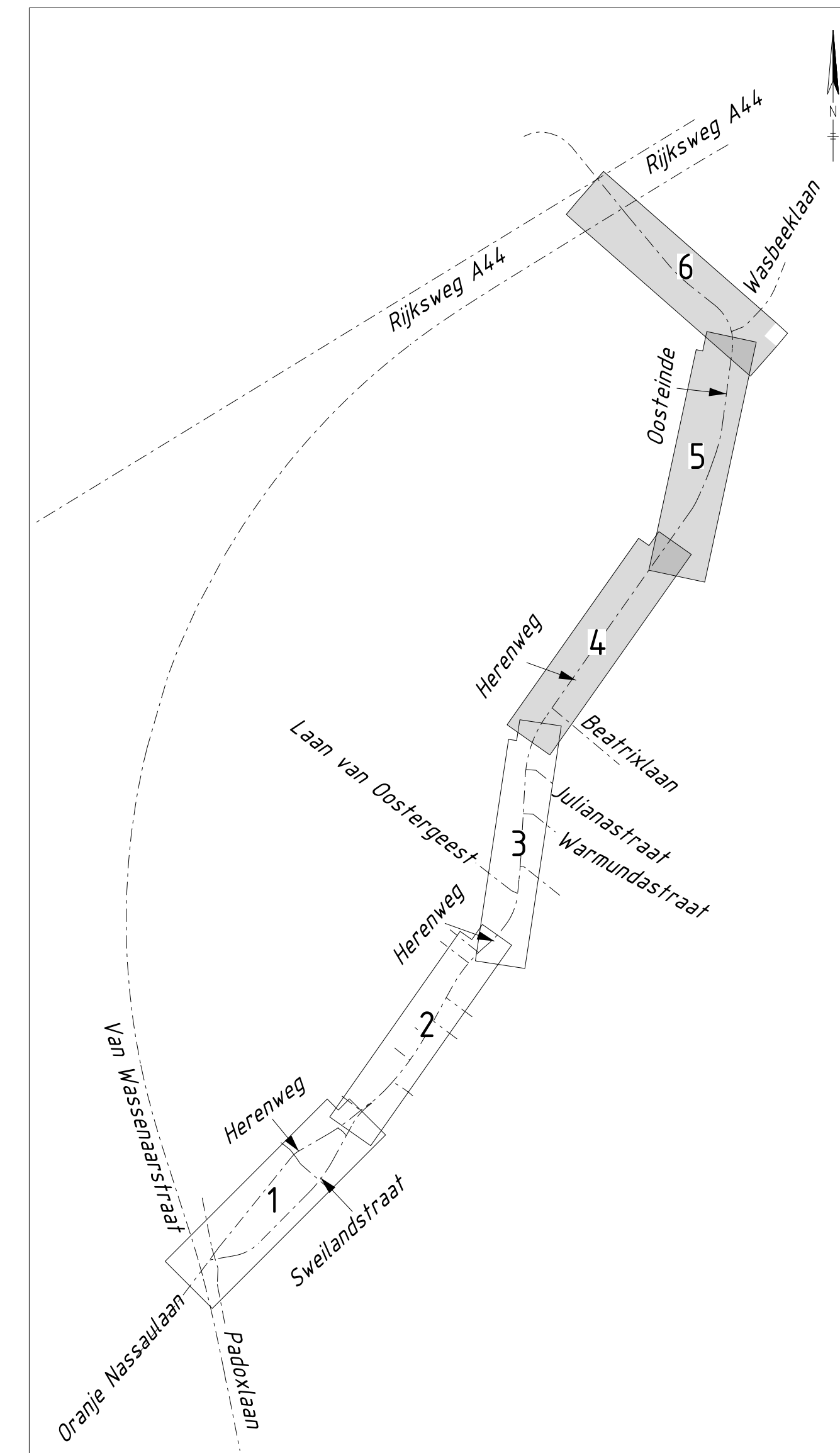
SITUATIE Schaal 1:10.000
